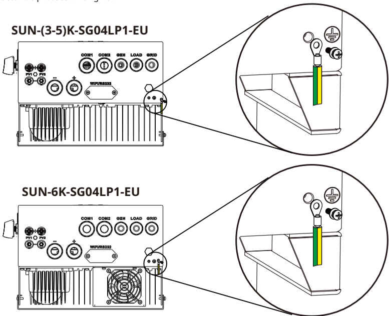
Conexión a tierra (cables de cobre)
