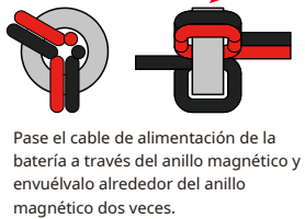
Entrada de batería de CC
