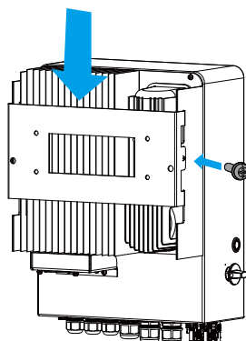
Instalación de la placa colgante del inversor
